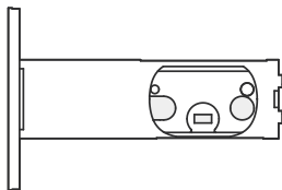
D 2-3/8" Backset
